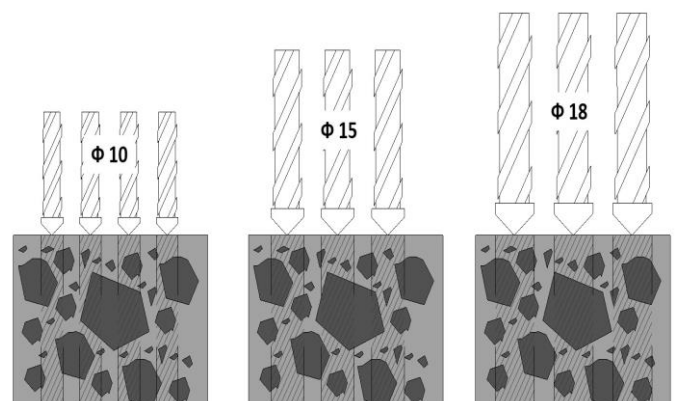
Figure 2. Model of drilling with a different diameter bits / schema di foratura con punte di diverso diametro
