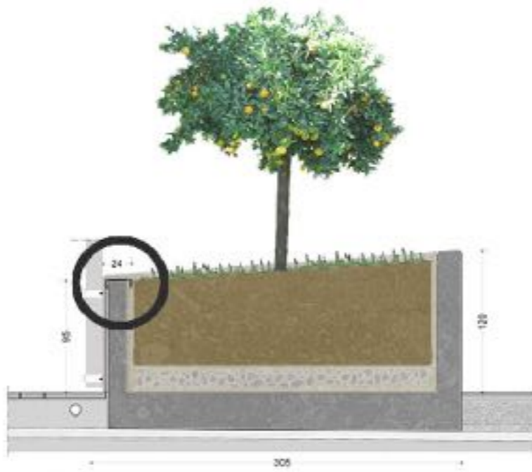
Sezione A-A
