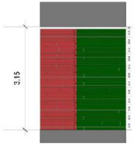
PROSPETTO E SEZIONE FASCIA 2
