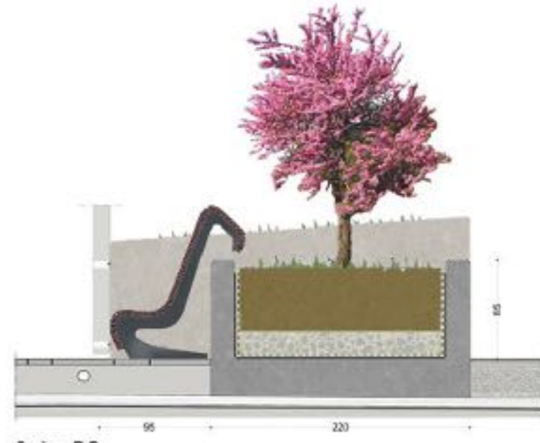
Sezione B-B
